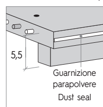
Particolare base con zoccolo Detail of base with plinth
