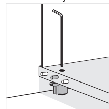
Particolare piedino regolabile. Detail of adjustable foot.
